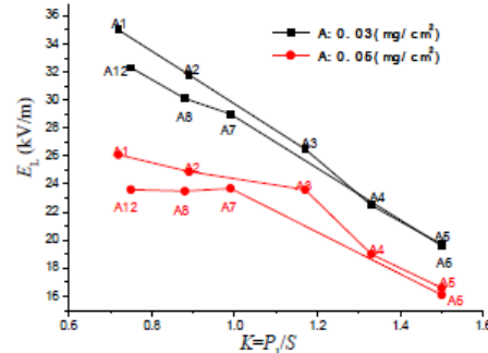
شکل (۲): رابطه بین E_L, K (ولتاژ جرقه برای هر واحد فاصله خزشی) [۷]
