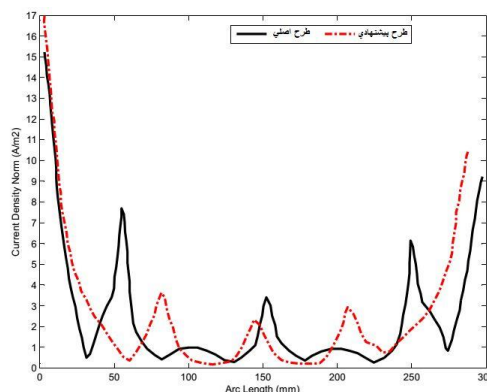
شکل (۶): دانسیته جریان ناشی در طرح اصلی و طرح پیشنهادی
