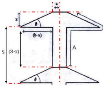
شکل (۱): هندسه پایه یک ایزولاتور پلیمری
