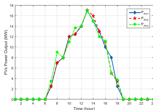
شکل (۵): توان خروجی مزارع خورشیدی مختلف در هر ساعت از سناریو ۱
