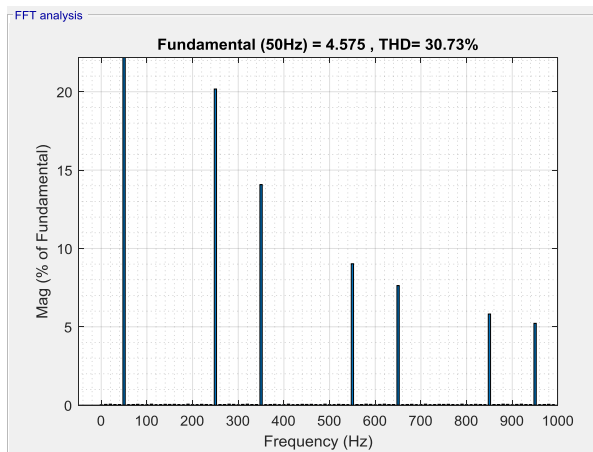
شکل (۱۴): مقدار THD جریان بار برای فاز A
