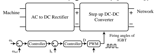
شکل (۳): بلوک دیاگرام کنترل مبدل بوست لینک DC
