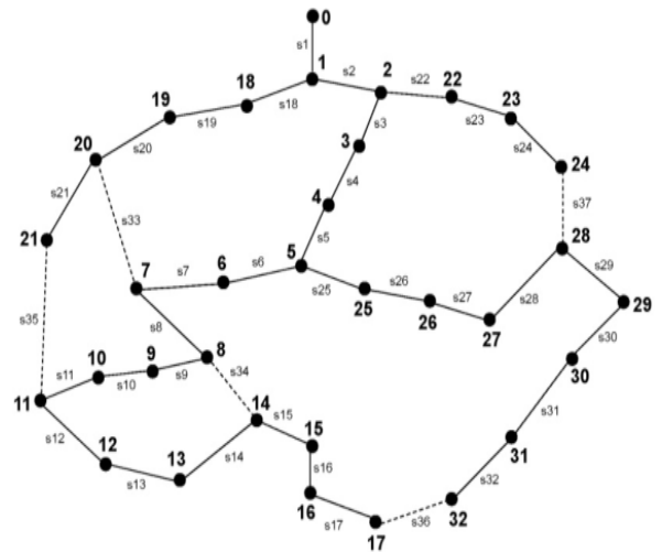
شکل ۲. دیگرام تک‌خطی شبکه آزمون ۳۲ شینه
