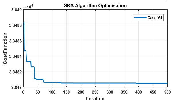
شکل (۷): رفتار همگرایی تابع هدف برای حالت (V.i) سیستم ۳ واحد
