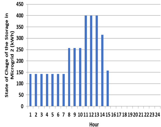
شکل (۱۳): وضعیت شارژ باتری‌های ذخیره انرژی در ریزشبه ۲
