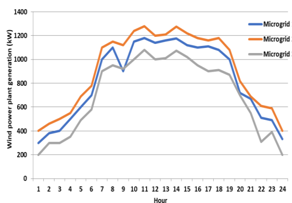
شکل (۶): تولید واحدهای بادی در ریز شبکه‌ها [۲۷]
