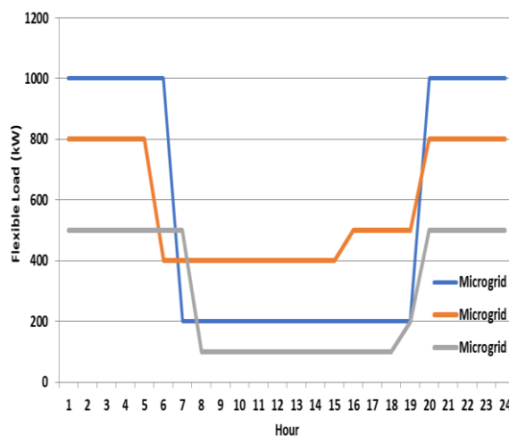
شکل (۵): بار قابل تنظیم در ریز شبکه‌ها
