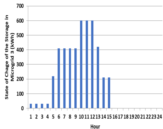
شکل (۱۴): وضعیت شارژ باتری‌های ذخیره انرژی در ریزشبه ۳
