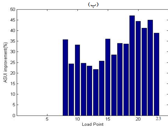
شکل (۲): چگونگی بهبود شاخص ASUI برای تک تک بارهای شبکه توزیع فعال نمونه: الف) مقایسه مقادیر متناظر ب) میزان برحسب درصد
