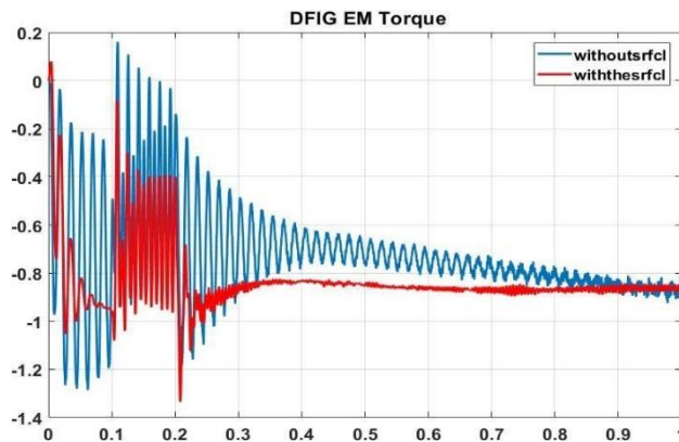
شکل (۱۵)- گشتاور ژنراتور القایی از دو سوتغذیه تحت خطای تکفاز
