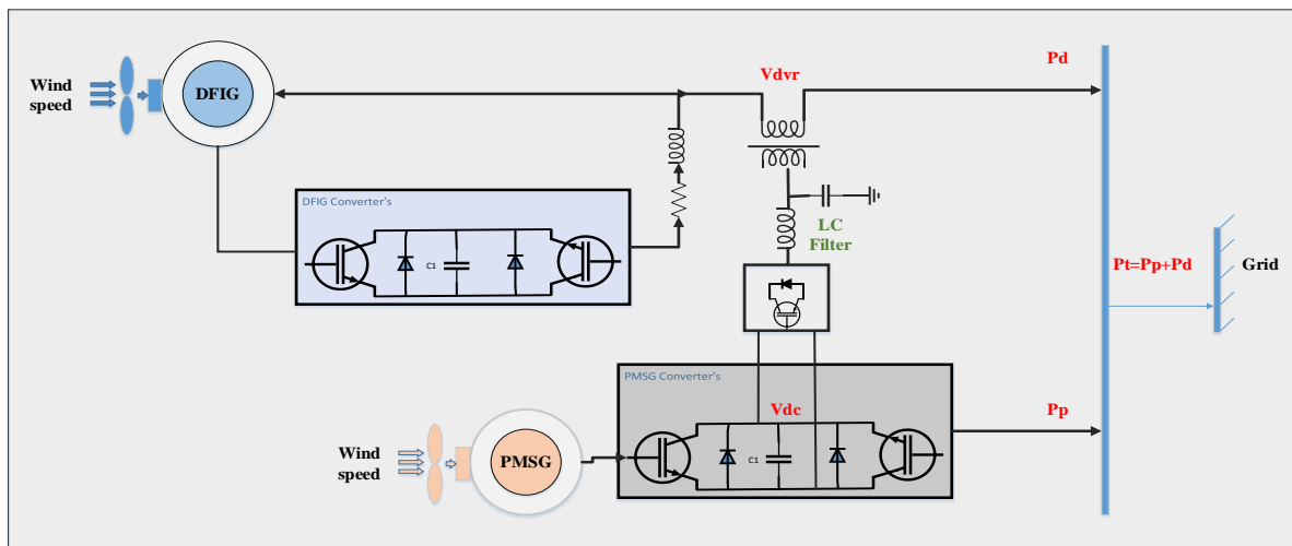
شکل (۱)- ساختار DFIG-WECS
