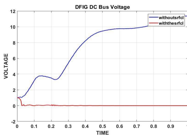
شکل (۲۴)-ولتاژ لینک dc ژنراتور القایی در شرایط باز شدن خط بعد از ژنراتور القایی
