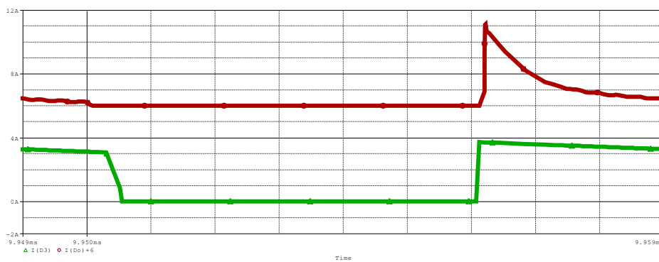
شکل (۹) شکل موج جریان دیودهای D3 و Do مدل شبیه سازی شده در مقیاس (1 \mu\text{s}/\text{div}, 1\text{A}/\text{div})
