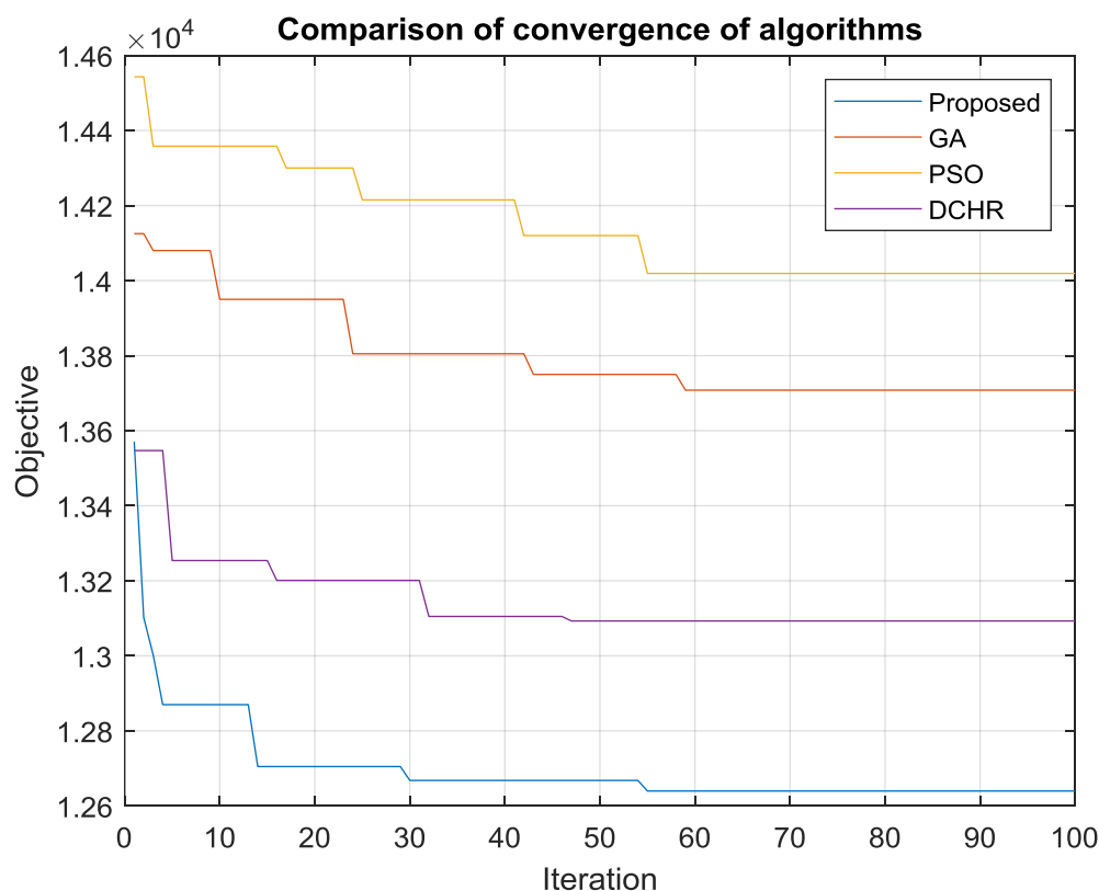
شکل (۳): مقایسه همگرایی الگوریتم‌ها Figure (3): Comparison of convergence of algorithms
