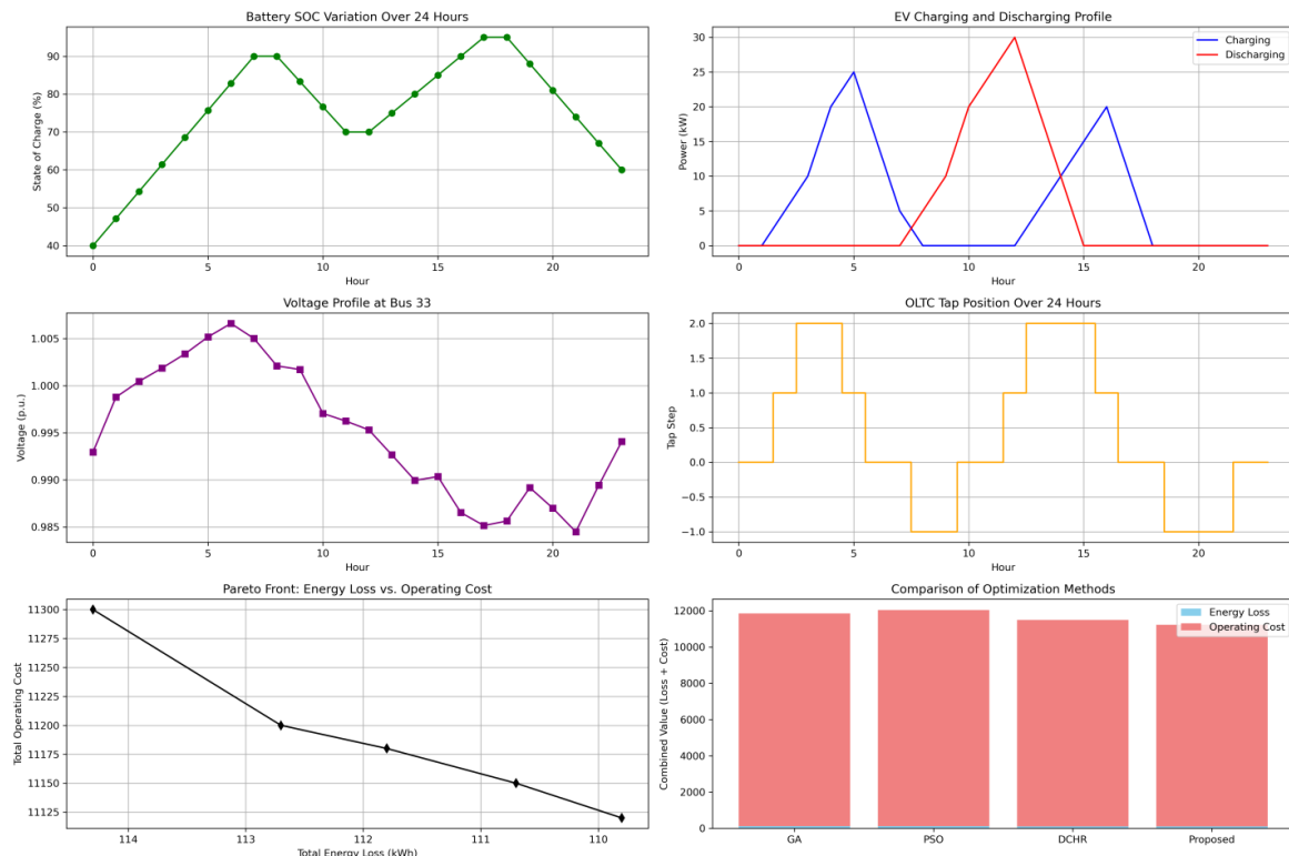
شکل (۲): نمودارهای تحلیلی مربوط به نتایج بهره‌برداری بهینه شبکه توزیع ۳۳ شینه تحت مدل پیشنهادی شامل الگوریتم فازی-ژنتیک و تجهیزات کنترلی هوشمند
