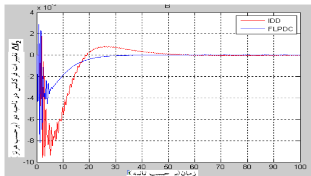
ب: تغییرات فرکانس در ناحیه ۲
