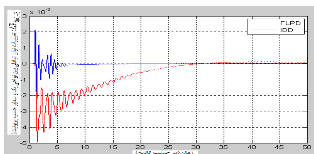
ت: تغییرات توان تبدالی بین نواحی ۱ و ۳
