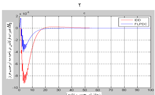
پ: تغییرات فرکانس در ناحیه ۳
