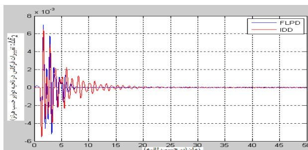
الف: تغییرات فرکانس در ناحیه ۲
