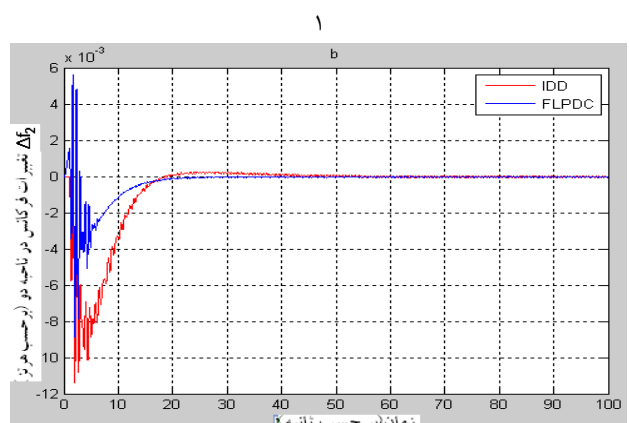
ب: تغییرات فرکانس در ناحیه
