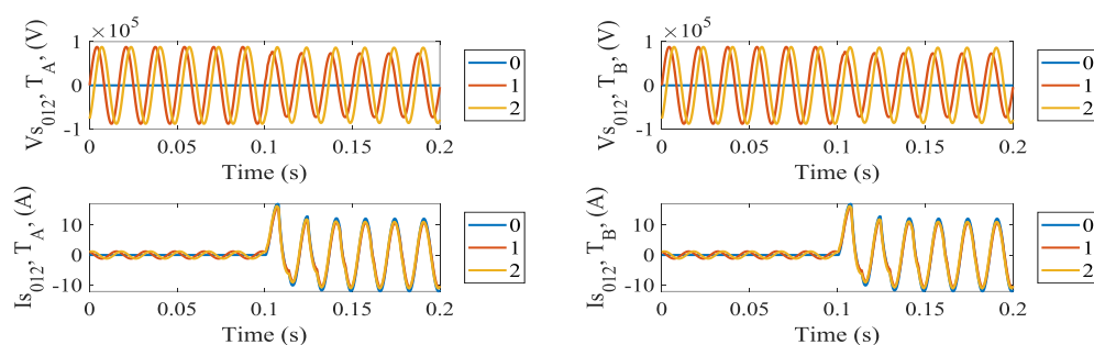
شکل (۱۰): ولتاژ و جریان مدل محاسبه شده برای سمت ثانویه ترانسفورماتورهای VT و CT روی ترمینال‌های A و B تحت خطای داخلی a-g
