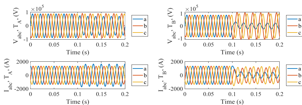
شکل (۱۱): ولتاژ و جریان سه‌فاز اندازه‌گیری شده روی ترمینال‌های A و B تحت خطای خارجی a-g
