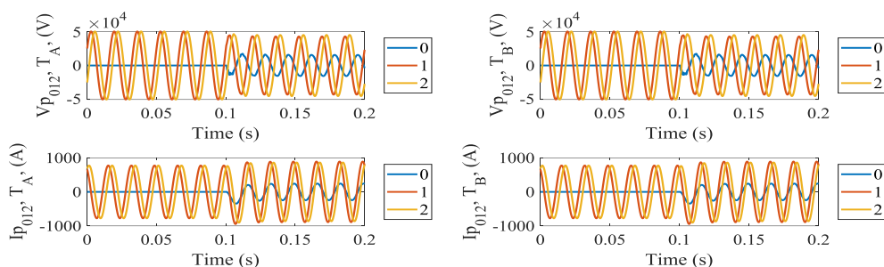
شکل (۹): ولتاژ و جریان مدل محاسبه شده برای سمت اولیه ترانسفورماتورهای VT و CT روی ترمینال‌های A و B تحت خطای داخلی a-g
