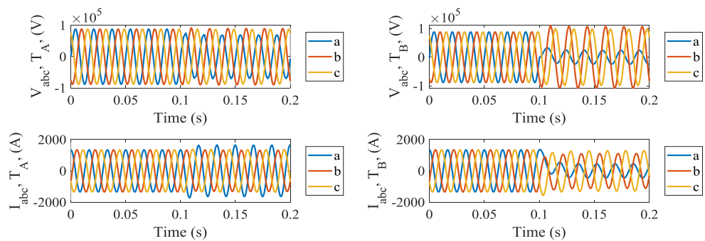
شکل (۱۱): ولتاژ و جریان سه‌فاز اندازه‌گیری شده روی ترمینال‌های A و B تحت خطای خارجی a-g Figure (11): Three-phase voltage and current measured on terminals A and B under external fault a-g
