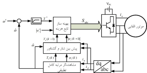
شکل ۲: ساختار کلی روش کنترل پیش بین شار بدون حسگر
