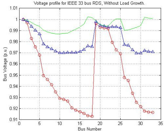
شکل (۴): پروفیل ولتاژ برای RDS ۳۳ شینه IEEE
