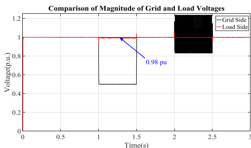
شکل (۱۵): دامنه ولتاژ سمت بار در سناریوی دوم
