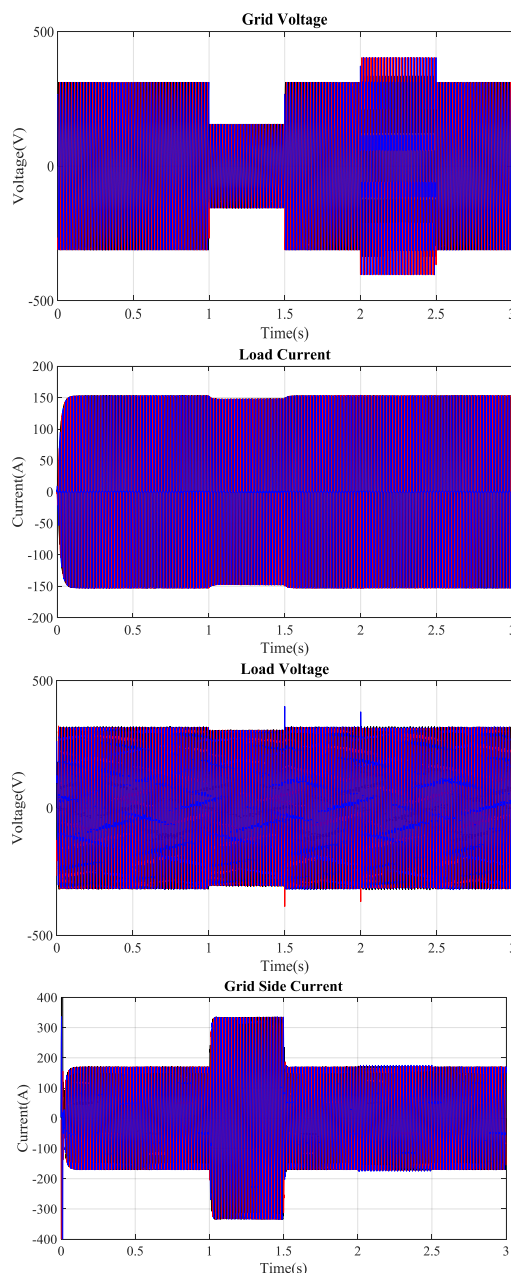
شکل (۹): نتایج شبیه‌سازی سناریوی اول
