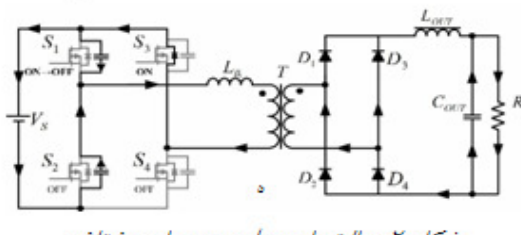
شکل ۲: حالت‌های مدار در مدهای مختلف
