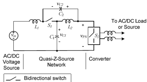
شکل (۳): ساختار کلی از یک مبدل شبه منبع امپدانس نوع تغذیه شده با منبع ولتاژ
