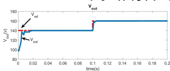
شکل (۸) ولتاژ خروجی کنترل کننده فازی و مرجع آن در حالت افزایش ولتاژ مرجع
