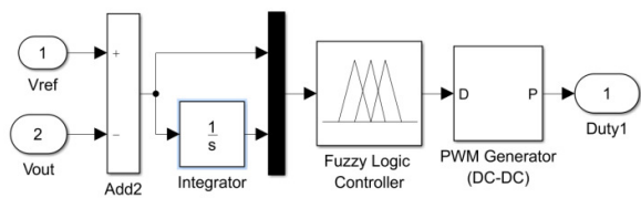
شکل (۷): بلوک دیاگرام بخش کنترل
