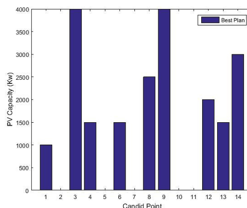
شکل (۷): ظرفیت‌های بهینه انتخاب شده برای منابع PV با در نظر گرفتن عدم قطعیت بار
