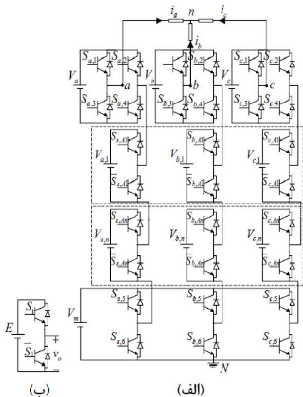
شکل (۲): الف) ساختار اینورتر چندسطحی مدولار ترکیبی (ب) ساختار سلول کمکی
