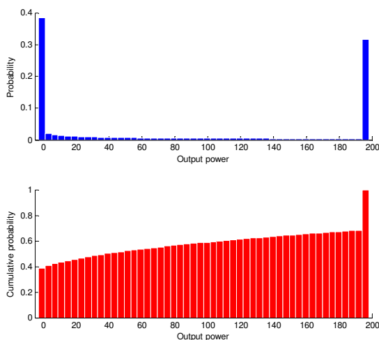
شکل (۴): احتمال تولید توان در توربین- ژنراتورهای بادی
