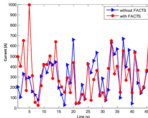
شکل (۸): جریان خطوط شبکه
