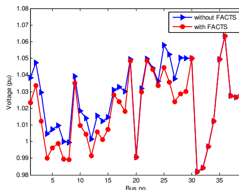
شکل (۱۱): پروفیل ولتاژ شین‌های شبکه در شرایط اضافه بار
