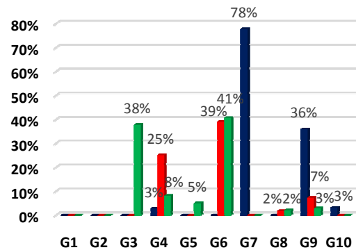
شکل(۴): درصد اختلاف تولید واحدها با در نظر گرفتن محدودیت سوخت و بدون آن بر مبنای پروپونیت
