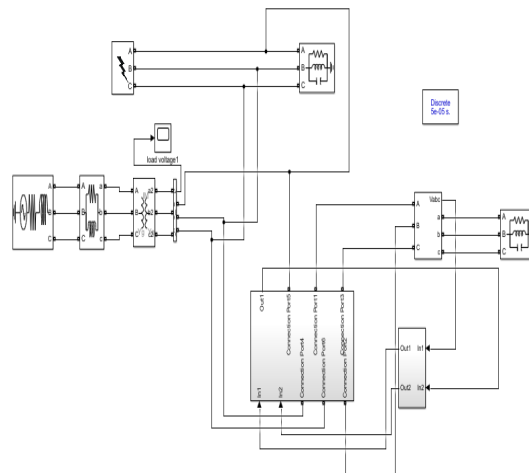
شکل (۲): مدار مورد مطالعه در این تحقیق
