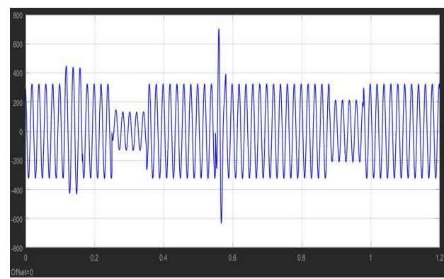
شکل (۹): موج خروجی فاز C در اثر ایجاد خطا، ورود و خروج بارهای مهمی، سلفی و خازنی
