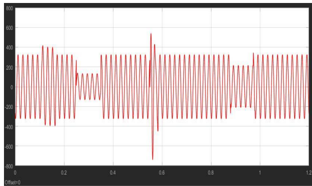
شکل (۸): موج خروجی فاز B در اثر ایجاد خطا، ورود و خروج بارهای مهمی، سلفی و خازنی
