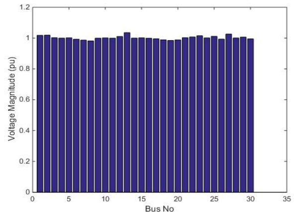
شکل (۷) نمودار اندازه ولتاژ با تابع پروفیل ولتاژ
