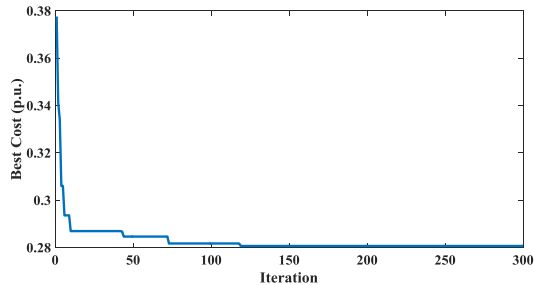
شکل (۹): منحنی همگرایی مربوط به الگوریتم ICA در فرآیند بازآرایی سیستم ۳۳ شینه با بار صنعتی
