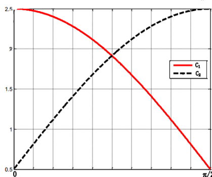
شکل (۱) ضرایب شتاب سینوس کسینوس [۵]
