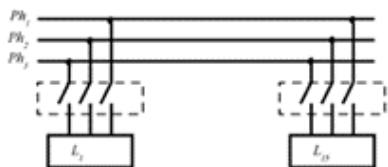
شکل (۱): نمونه فیدر توزیع
