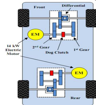
شکل (۶): لایه بندی تجهیزات نیرومحرکه
