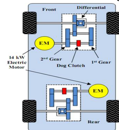
شکل (۶): لایه بندی تجهیزات نیرومحرکه
