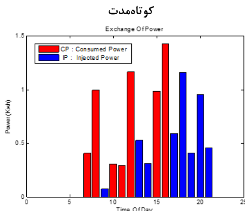
شکل (۹): تبادل توان با شبکه در حالت شارژ کند - بازه زمانی بلندمدت
