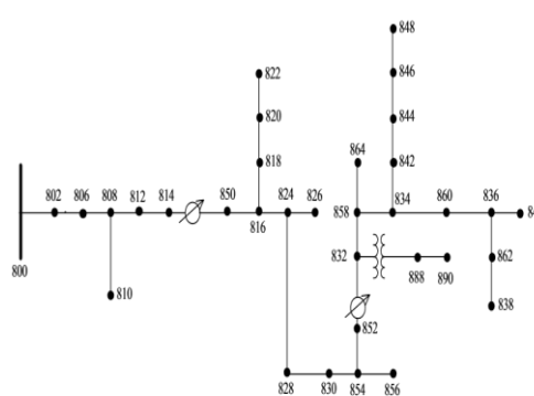
شکل (۱۱): شبکه استاندارد ۳۴ باس [۱۷]
