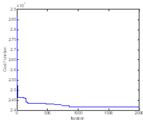
شکل (۵): نمودار همگرایی الگوریتم VCPSO را برای یافتن تابع هزینهی سیستم ۱۳ واحد با بار ۲۵۲۰ MW
