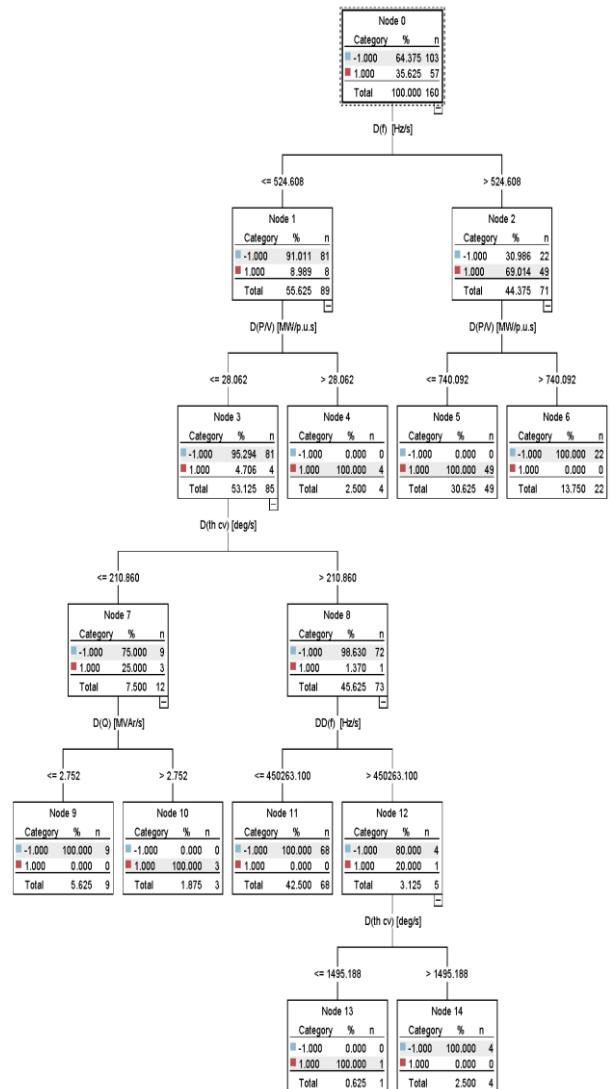
شکل (۶): درخت تصمیم آموزش دیده برای ریزش شبکه توسط داده های خاص اضافه شده با استفاده از اطلاعات باس سیستم فتوولتاییک
