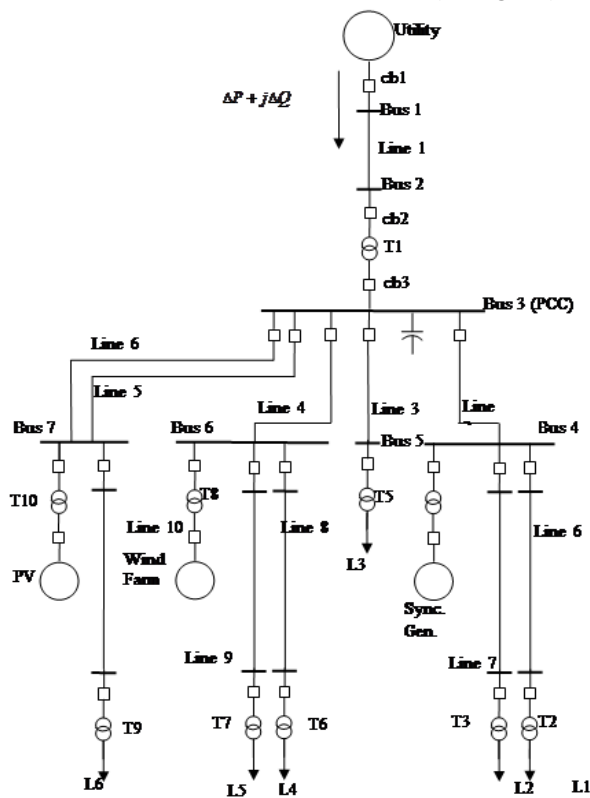
شکل (۱): سیستم توزیع مورد مطالعه
