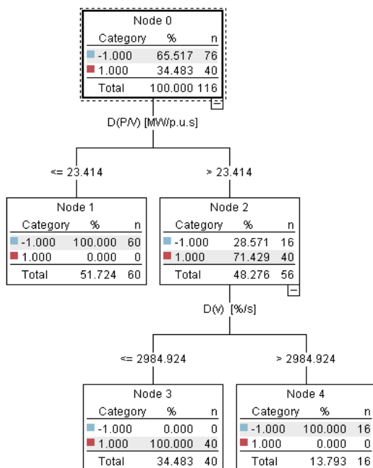
شکل (۴): درخت تصمیم مربوط به ریزش شبکه با استفاده از اطلاعات باس مولد فتوولتاییک
