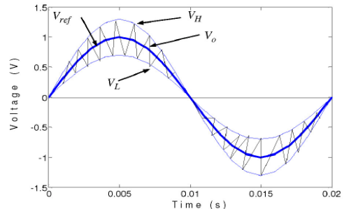
شکل (۸): اساس کار کنترلر ولتاژ هیستریزس [۳۲]
