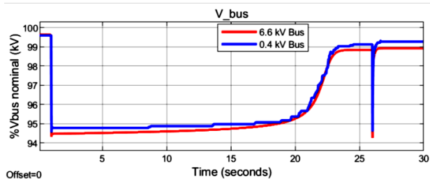
شکل ۱۶: ولتاژ باس‌های 0.4kV و 6.6kV در راه اندازی با اتوترانسفورماتور
