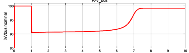
شکل ۸: شبیه‌سازی رفتار دینامیکی موتور القایی با روش DOL به همراه فیدرهای 0.4kV و 6.6kV
