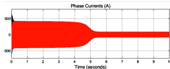
شکل ۳: جریان راه اندازی موتور با روش DOL
