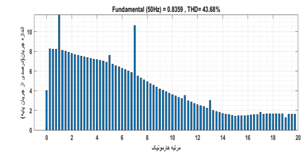
شکل (۷): اعوجاج‌های هارمونیک کل جریان سمت شبکه در حالت بدون فیلتر
