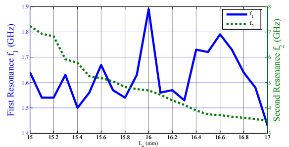
شکل (۸): تغییر محل فرکانس های تشدید به ازای تغییرات L_6
