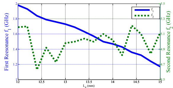
شکل (۷): تغییر محل فرکانس های تشدید به ازای تغییرات L_4
