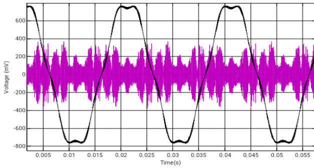
شکل ۵: ولتاژ تخلیه جزئی در قسمت پوشش خازن قدرت
