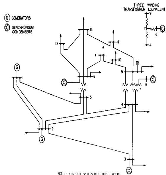
شکل (۵): شبکه ۱۴ شینه IEEE پس از خروج خط
