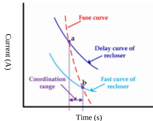
شکل (۲): مشخصه جریان-زمان برای بررسی هماهنگی حفاظتی براساس طرح حفظ فیوز
