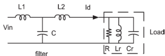
شکل (۸): فیلتر LCL و بار موازی [8]
