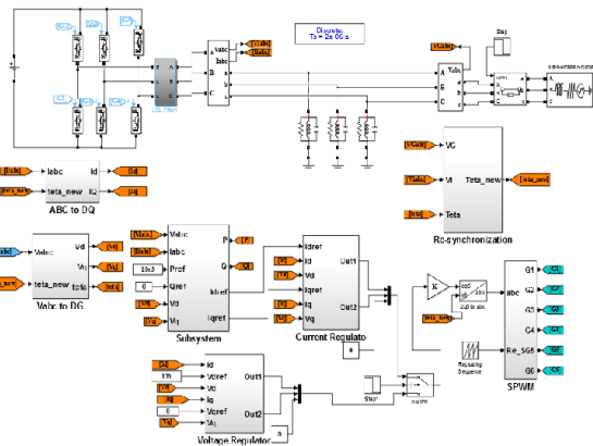
شکل (۱۱): مدل شبیه‌سازی DG و سیستم کنترل
