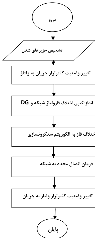
شکل (۱۰): فلوجارت الگوریتم پیشنهادی
