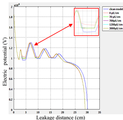
شکل (۱۴): فاصله نشت پتانسیل الکتریکی برای رسانایی های مختلف [۴۹-۵۰]
