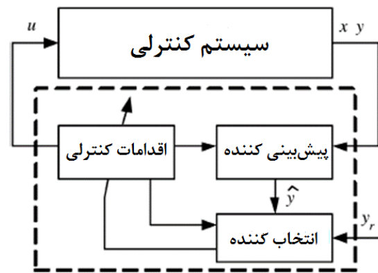
شکل (۳): اجزای مدل کنترل مبتنی بر پیش‌بین [۵]
