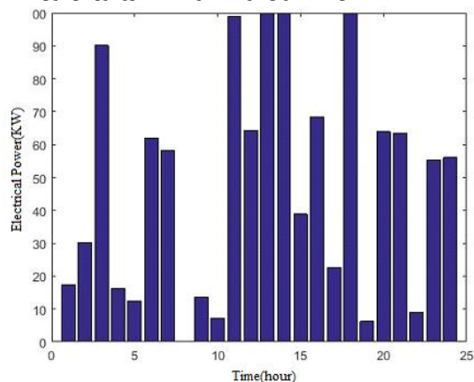
شکل (۹): توان تولیدی واحد میکرو توربین دوم
