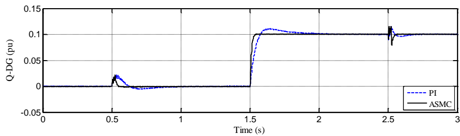
شکل (۴): توان راکتیو DG برحسب پریونیت
